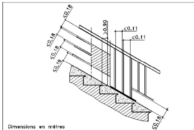
escalier à limon
